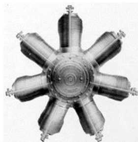
Motor Gnome 50 CV.
