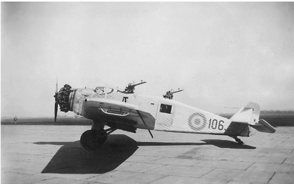
Junker K -43 N° 106 mostrando todo su armamento. Dos ametralladoras Madsen de 7,65 mm en torretas giratorias y bombas bajo sus planos.
